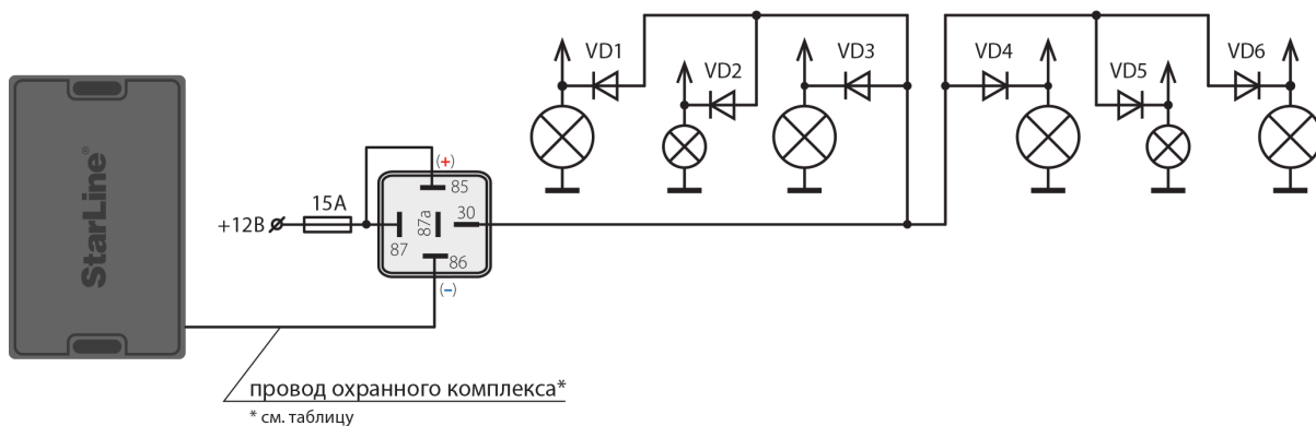
Подключение световых сигналов для охранных комплексов E96/66, S96/66, M96
